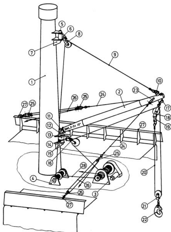
Slika 1.3.8.2 Teška samarica
