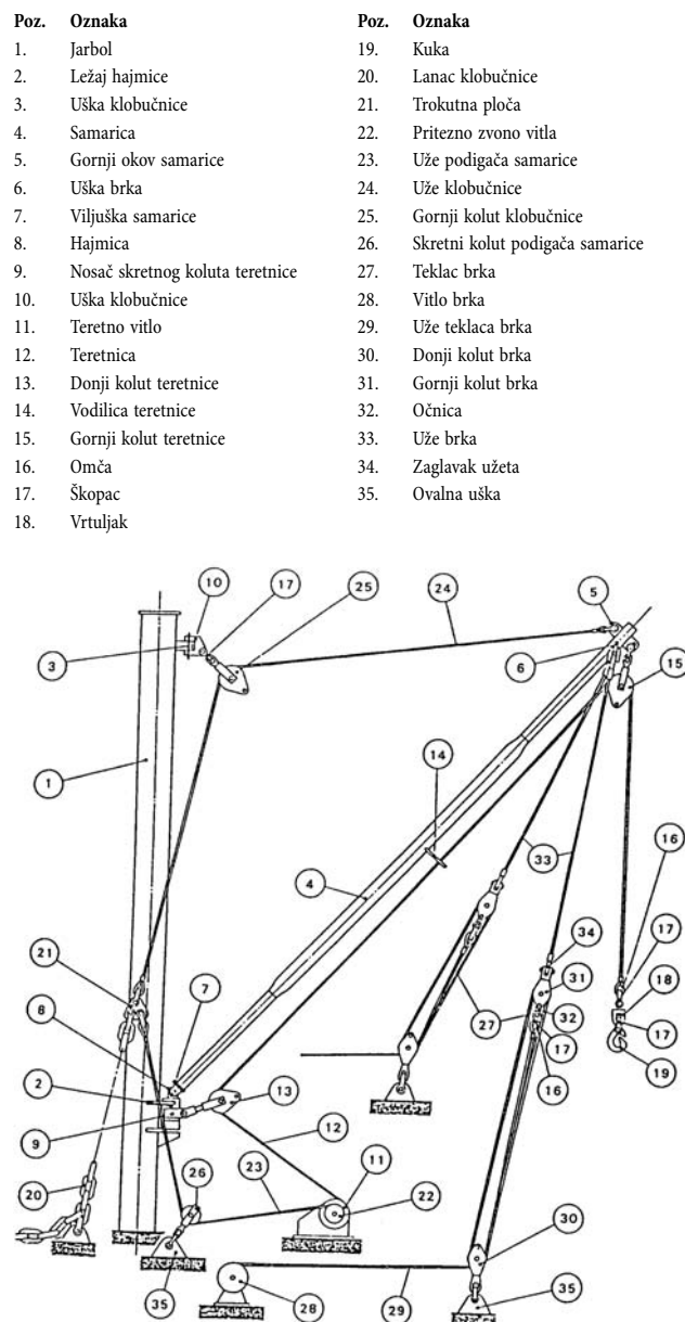
Slika 1.3.8.1 Laka samarica
