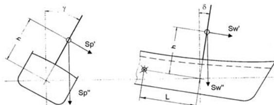
Ljudljanje broda
