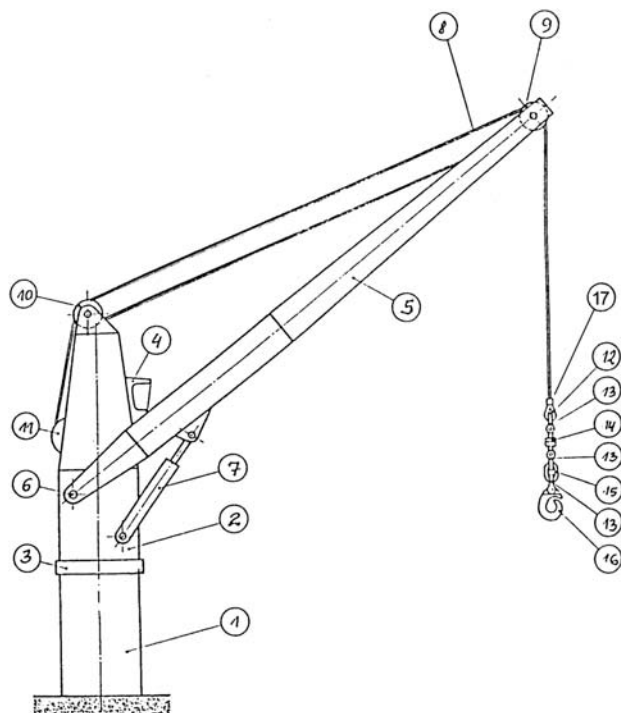
Slika 1.3.8.5 Palubna dizalica
