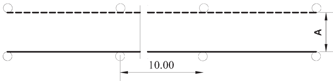
Слика 27. Простор и ознаке простора за извођење полигонске радње „вожња напред са променом степена преноса и уназад у истој саобраћајној траци” (за оспособљавање кандидата за возаче моторних возила категорије М)
