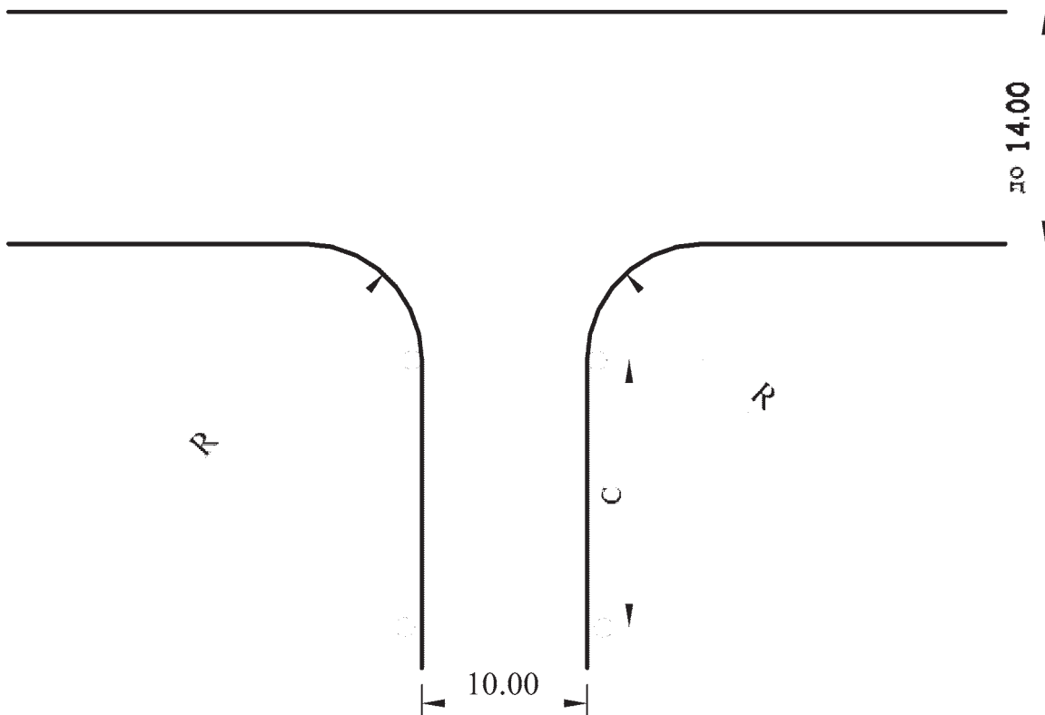
Слика 22. Простор и ознаке простора за извођење полигонске радње „вожња напред са променом степена преноса и уназад у истој саобраћајној траци” (за оспособљавање кандидата за возаче возила категорија D1E и DE)
