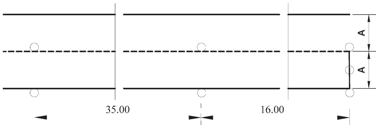
Слика 10. Простор и ознаке простора за извођење полигонске радње „кочење и заустављање” (за оспособљавање кандидата за возаче моторних возила категорија B1 и B)
