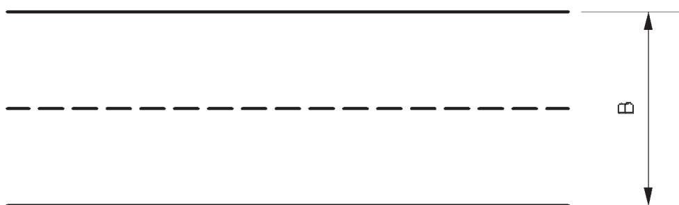
Слика 7. Простор и ознаке простора за извођење полигонске радње „паркирање возила под правим углом, вожњом уназад” (за оспособљавање кандидата за возаче моторних возила категорија B1 и B)
