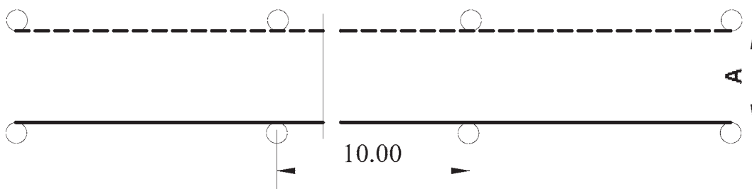
Слика 25. Простор и ознаке простора за извођење полигонске радње „вожња напред са променом степена преноса и уназад у истој саобраћајној траци” (за оспособљавање кандидата за возаче возила категорије F)
