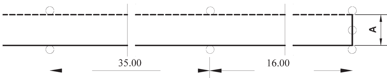
Слика 27. Простор и ознаке простора за извођење полигонске радње „вожња напред са променом степена преноса и уназад у истој саобраћајној траци” (за оспособљавање кандидата за возаче моторних возила категорије М)
