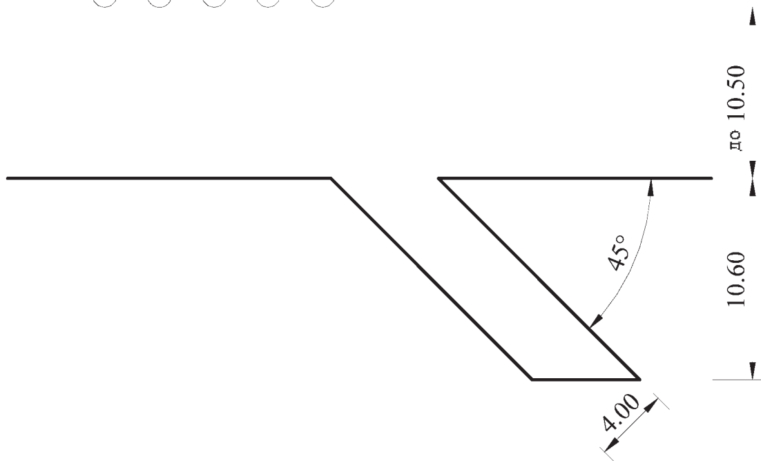
Слика 19. Простор и ознаке простора за извођење полигонске радње „заустављање возила на перону, ради изласка и уласка путника и полазак са перона” (за оспособљавање кандидата за возаче моторних возила категорија D1 и D)
