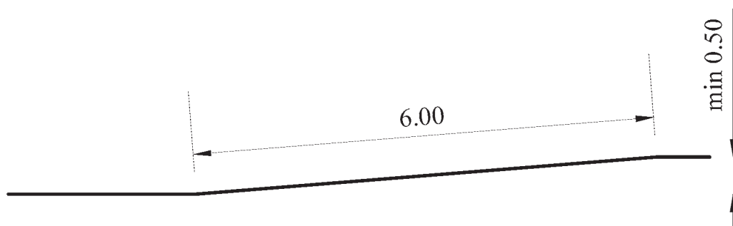
Слика 9. Простор и ознаке простора за извођење полигонске радње „заустављање и полазак возилом на путу са успоном” (за оспособљавање кандидата за возаче моторних возила категорија B1 и B)
