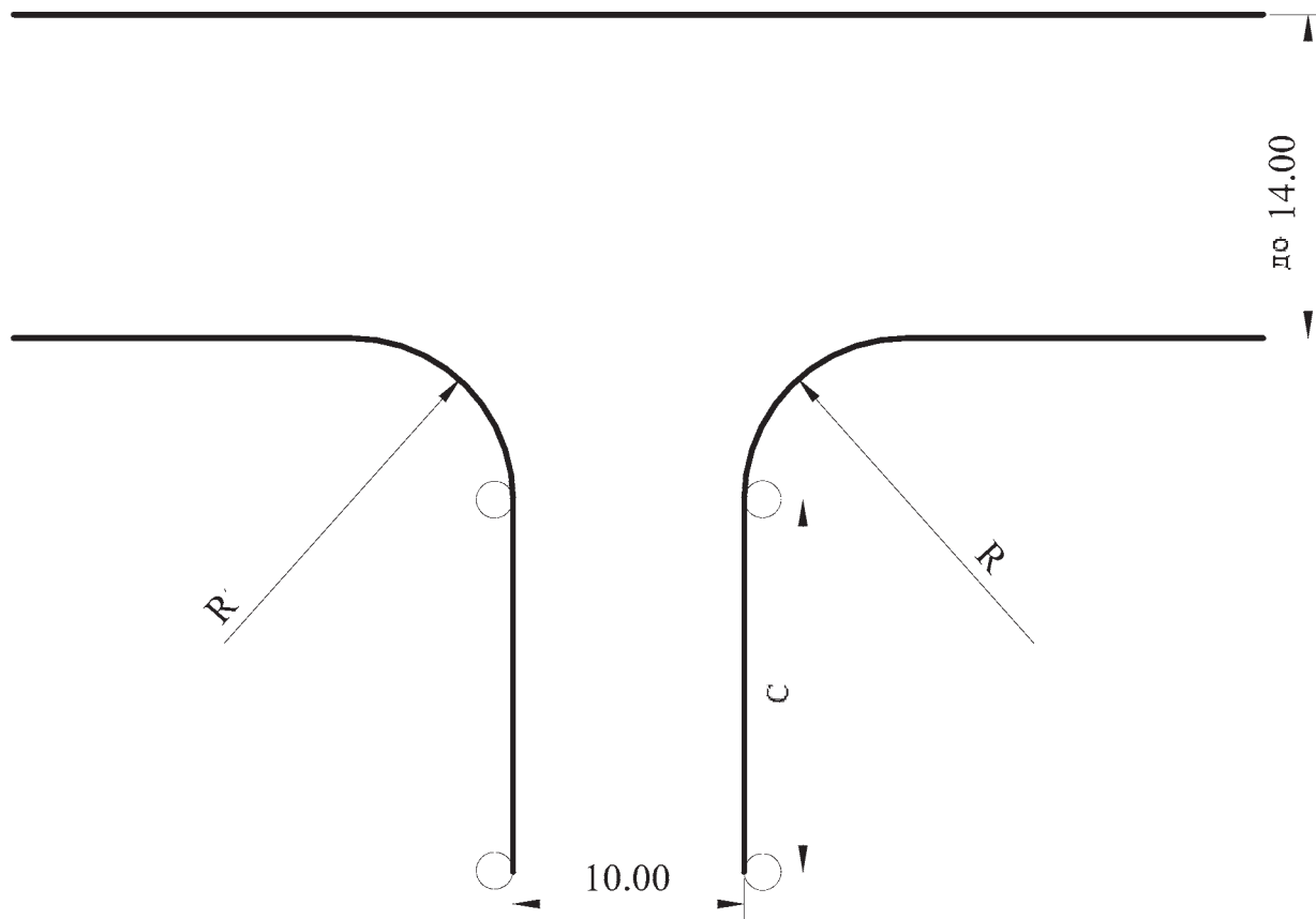
Слика 17. Простор и ознаке простора за извођење полигонске радње „вожња напред са променом степена преноса и уназад у истој саобраћајној траци” (за оспособљавање кандидата за возаче возила категорија C1E и CE)
