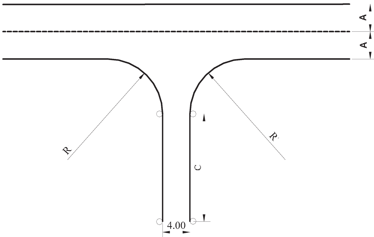
Слика 25. Простор и ознаке простора за извођење полигонске радње „вожња напред са променом степена преноса и уназад у истој саобраћајној траци” (за оспособљавање кандидата за возаче возила категорије F)
