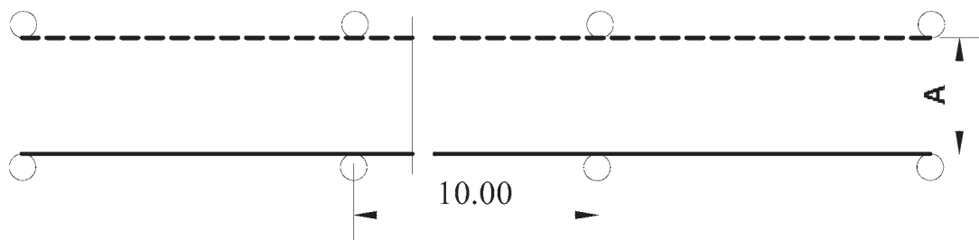
Слика 17. Простор и ознаке простора за извођење полигонске радње „вожња напред са променом степена преноса и уназад у истој саобраћајној траци” (за оспособљавање кандидата за возаче возила категорија C1E и CE)
