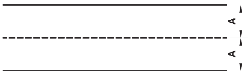
Слика 10. Простор и ознаке простора за извођење полигонске радње „кочење и заустављање” (за оспособљавање кандидата за возаче моторних возила категорија B1 и B)
