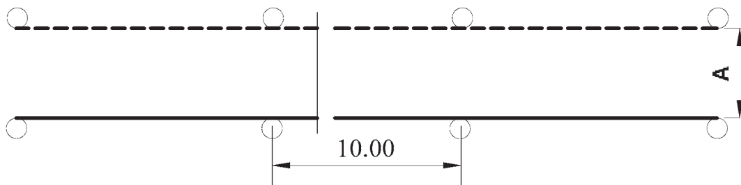
Слика 22. Простор и ознаке простора за извођење полигонске радње „вожња напред са променом степена преноса и уназад у истој саобраћајној траци” (за оспособљавање кандидата за возаче возила категорија D1E и DE)
