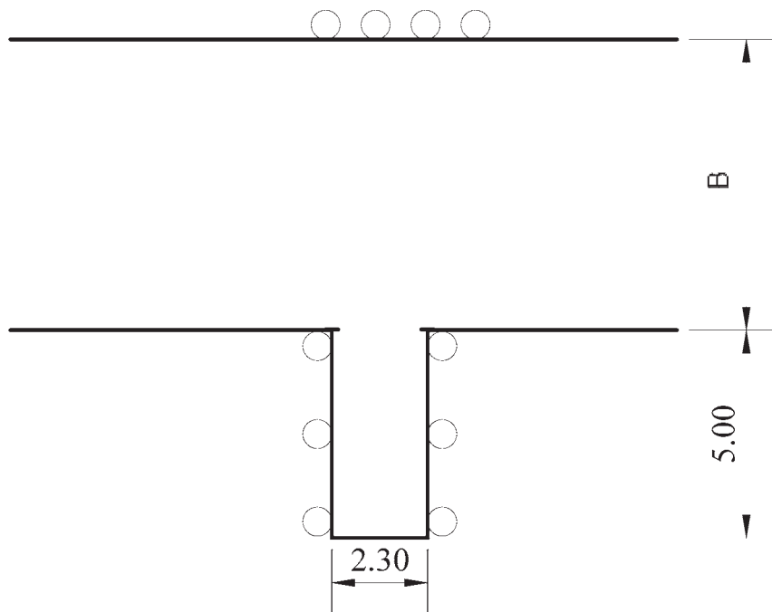
Слика 7. Простор и ознаке простора за извођење полигонске радње „паркирање возила под правим углом, вожњом уназад” (за оспособљавање кандидата за возаче моторних возила категорија B1 и B)
