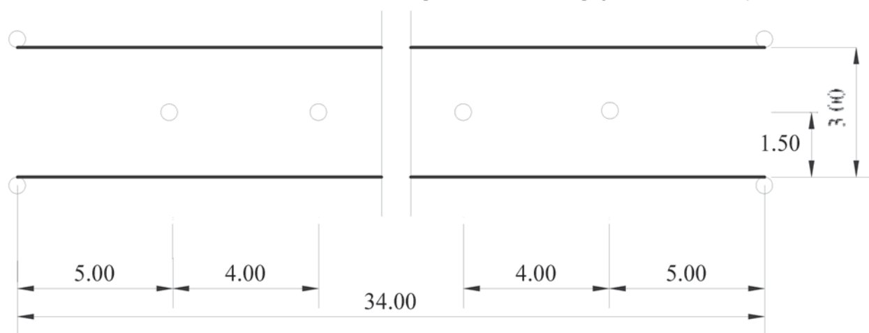
Слика 2. Простор и ознаке простора за извођење полигонске радње „слалом вожња” (за оспособљавање кандидата за возаче моторних возила категорија АМ, А1, А2 и А)
