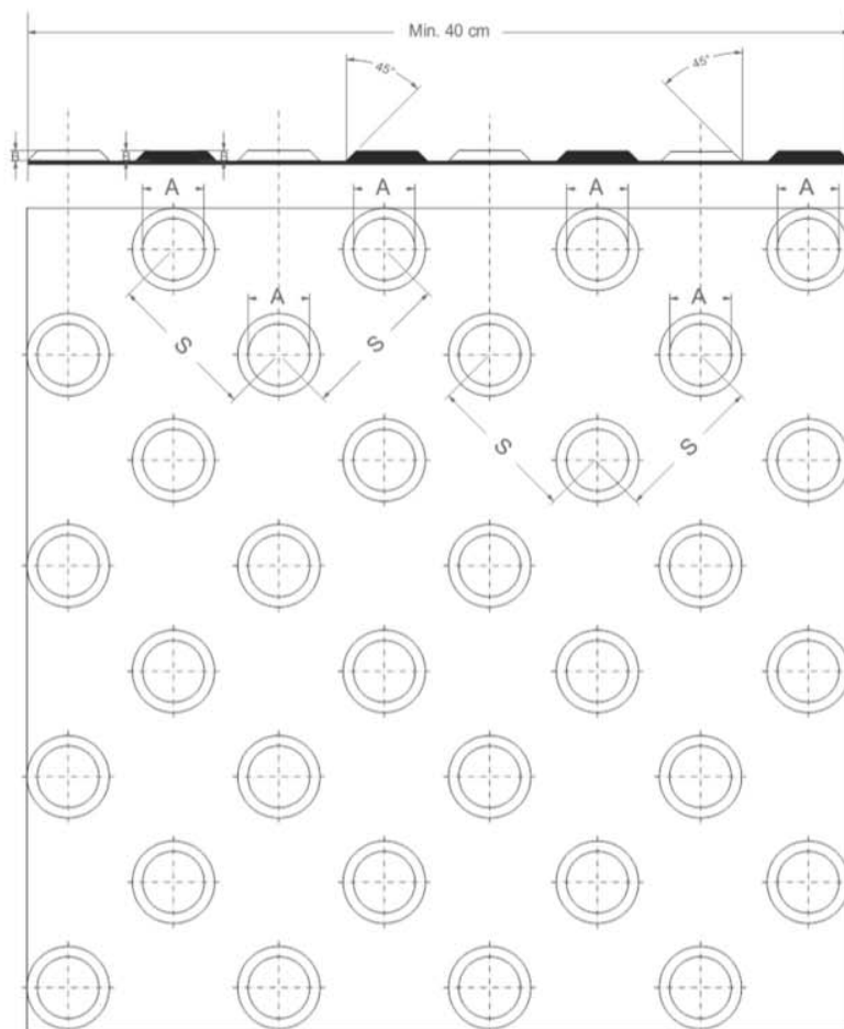
Слика 3.3 Дезен тактилног поља упозорења
