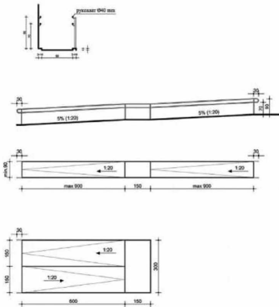
Слика 4. Рампе за пешаке
