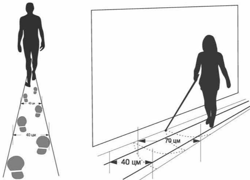
Слика 3.1.Ширина тактилних стаза
