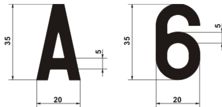
Slika 8. Dimenzije slovnih i brojčanih oznaka na registarskim tablicama za motocikl i teški tricikl
