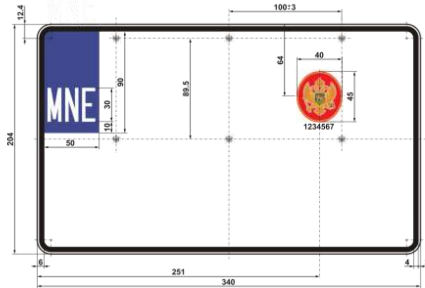
Slika 2. Izgled registarske tablice dimenzija 340 x 204 mm
