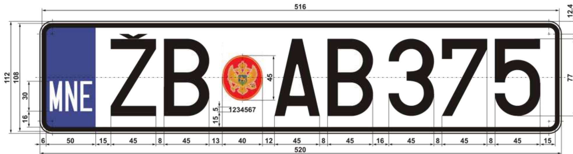
Slika 10.1. Registarska tablica za motorno vozilo
