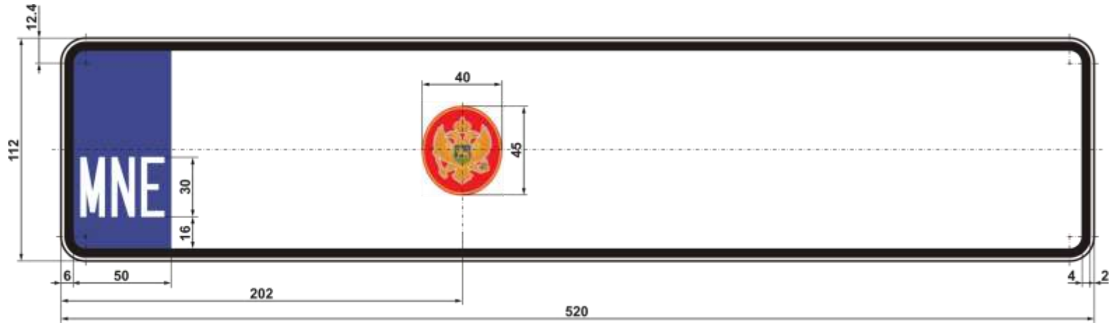
Slika 1. Izgled registarske tablice dimenzija 520 x 112 mm
