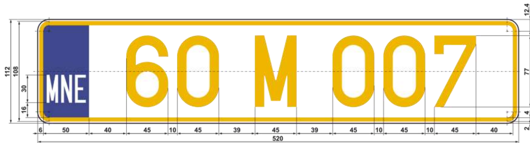
Slika 21. Registarska tablica za motorno vozilo stranaca zaposlenih u predstavništvima međunarodnih organizacija
