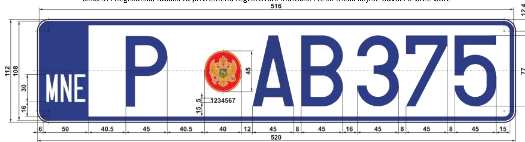
Slika 38. Registaraska tablica za motorno policijsko vozilo
