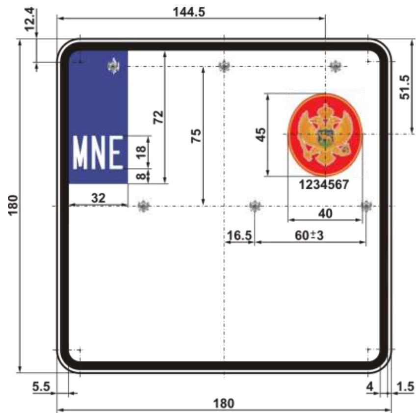
Slika 3. Izgled registarske tablice dimenzija 180 x 180 mm
