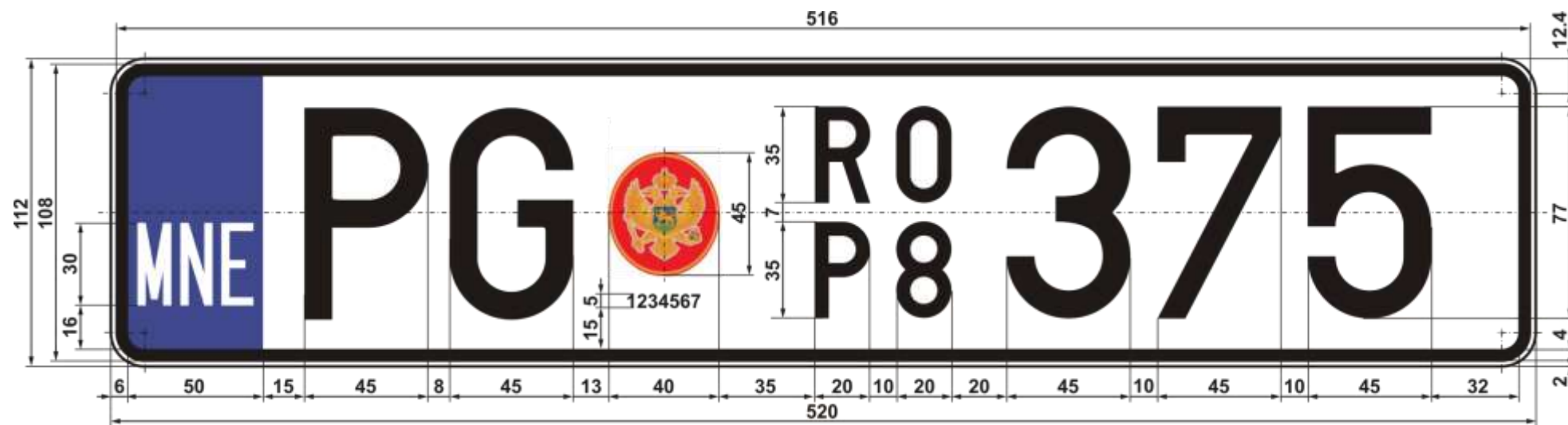
Slika 32. Registarska tablica za privremeno registrovano motorno vozilo
