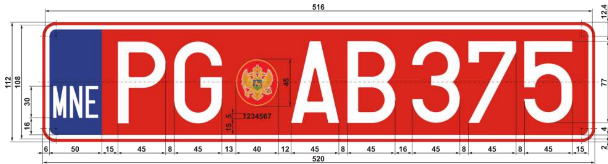
Slika 41. Registarska tablica za motorno vozilo koje ne ispunjava propisane uslove
