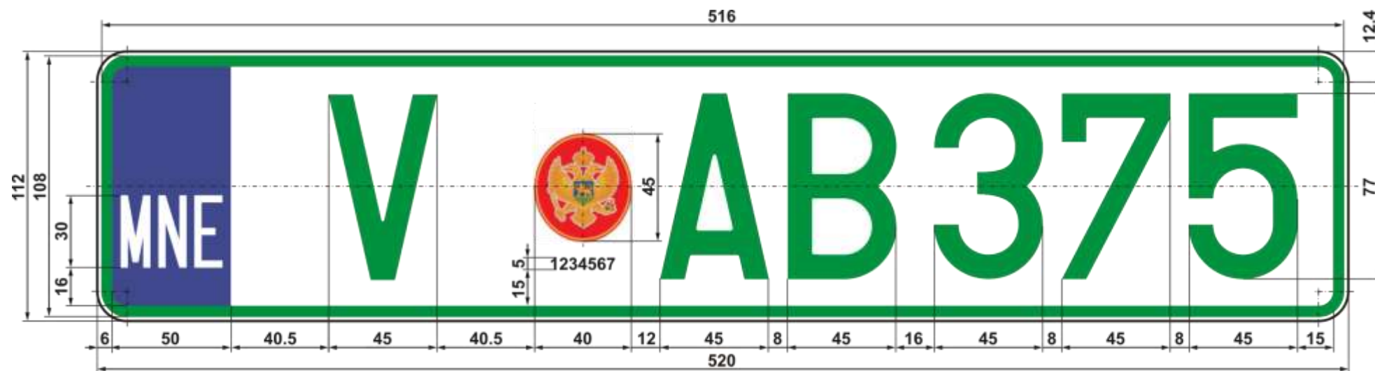
Slika 29. Registarska tablica za motorno vozilo Vojske Crne Gore
