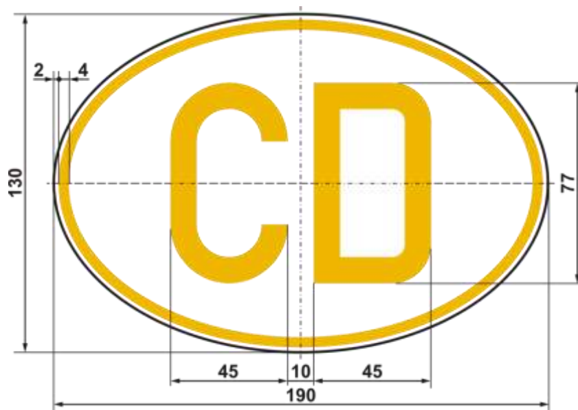
Slika 23. Dopunska tablica za vozilo lica sa diplomatskim statusom
