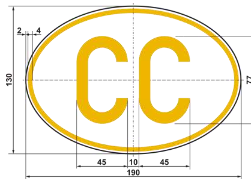
Slika 24. Dopunska tablica za vozilo konzularnih predstavništava ili lica sa konzularnim statusom
