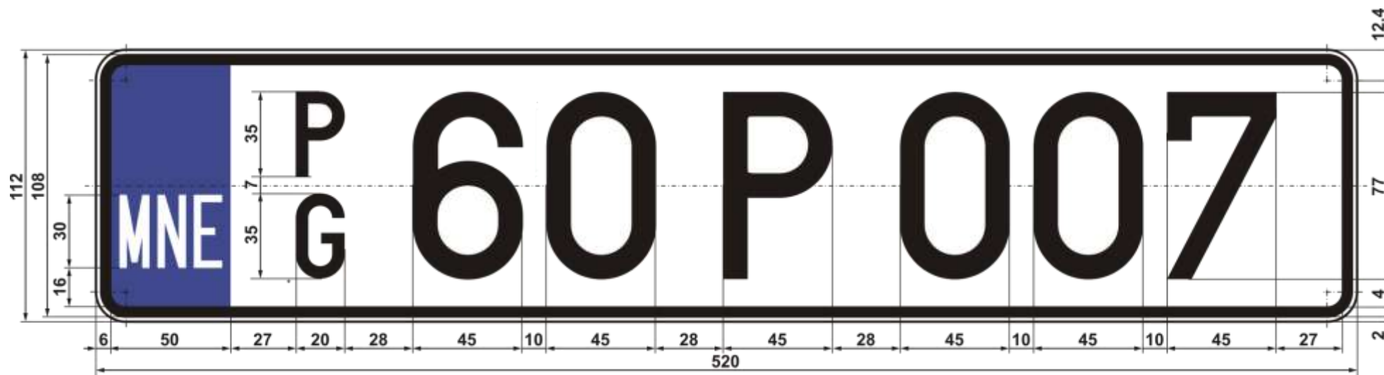
Slika 26. Registaraska tablica za motorno vozilo stranih trgovinskih, saobraćajnih, kulturnih i drugih predstavništava i stranih dopisništava
