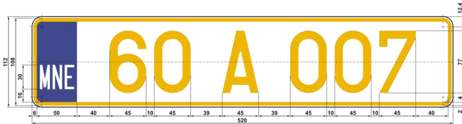
Slika 19. Registarska tablica za motorno vozilo diplomatskih predstavništava i misija stranih država i predstavništava međunarodnih organizacija i njihovog osoblja koje ima diplomatski status
