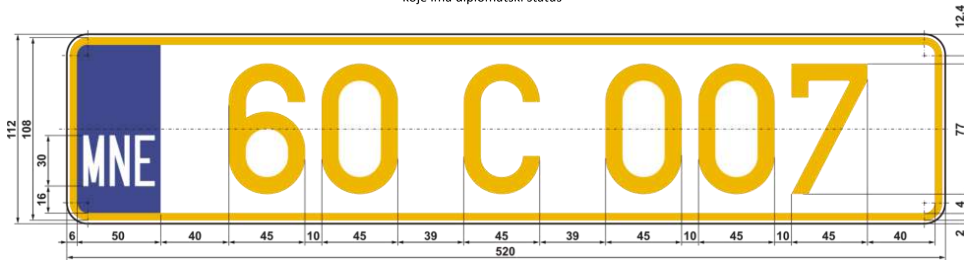
Slika 20. Registarska tablica za motorno vozilo konzularnih predstavništava i njihovog osoblja koje ima konzularni status
