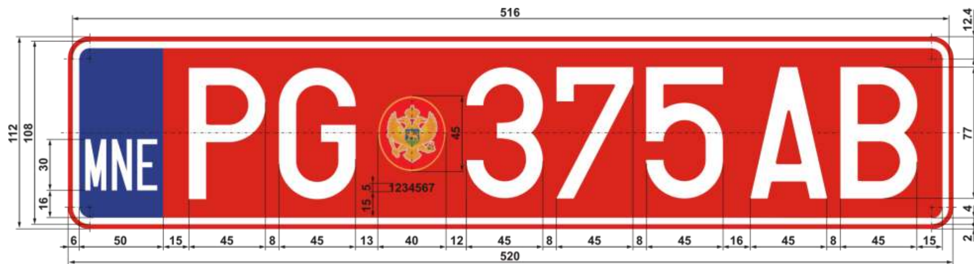
Slika 42. Registarska tablica za priključno vozilo koje ne ispunjava propisane uslove
