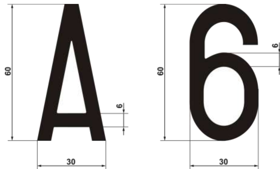
Slika 7. Dimenzije slovnih i brojčanih oznaka na registarskim tablicama za motocikl i teški tricikl
