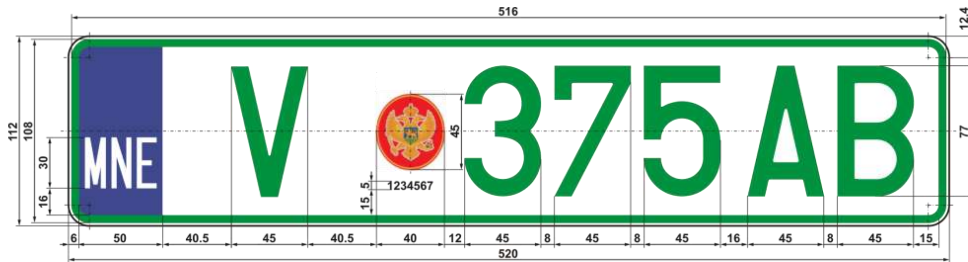
Slika 30. Registarska tablica za priključno vozilo Vojske Crne Gore
