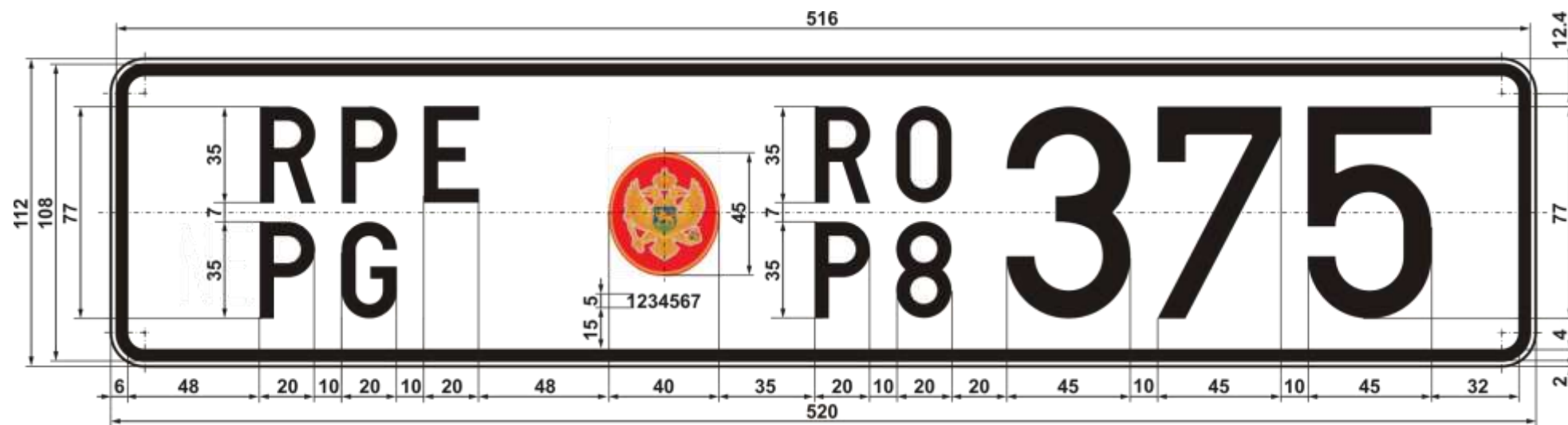
Slika 35. Registarska tablica za privremeno registrovano motorno vozilo koje se odvozi iz Crne Gore
