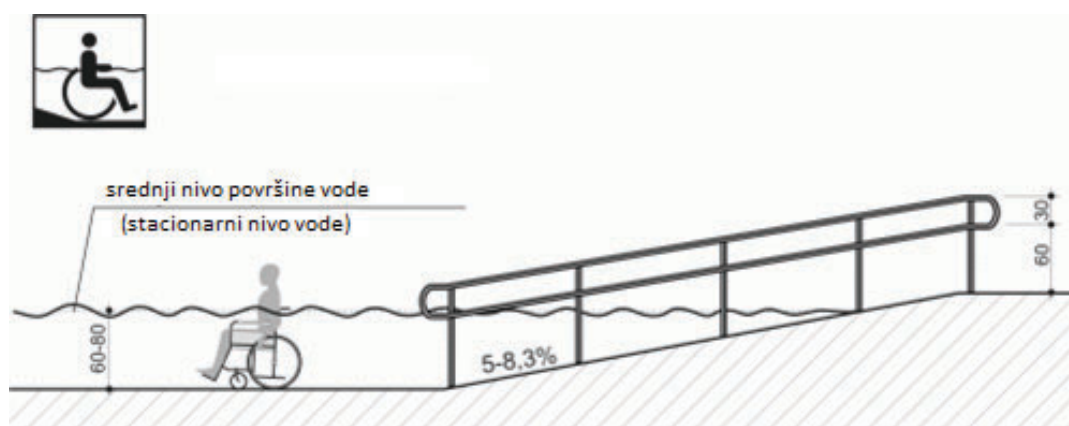
GRAFIČKI PRIKAZ BR. 27 - ULAZ U VODU
