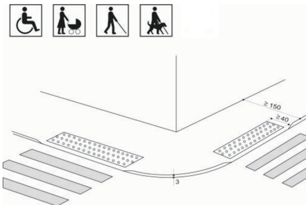
GRAFIČKI PRIKAZ BR. 37 - PJEŠAČKI PRELAZ NA MJESTU NAJMANJE VISINE TROTOARA
