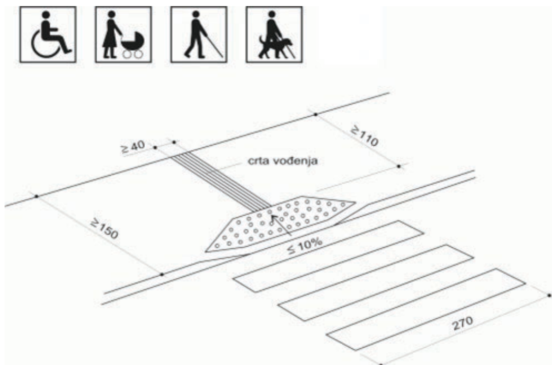
GRAFIČKI PRIKAZ BR. 38 - PJEŠAČKI PRELAZ IZVAN UKRŠTANJA
