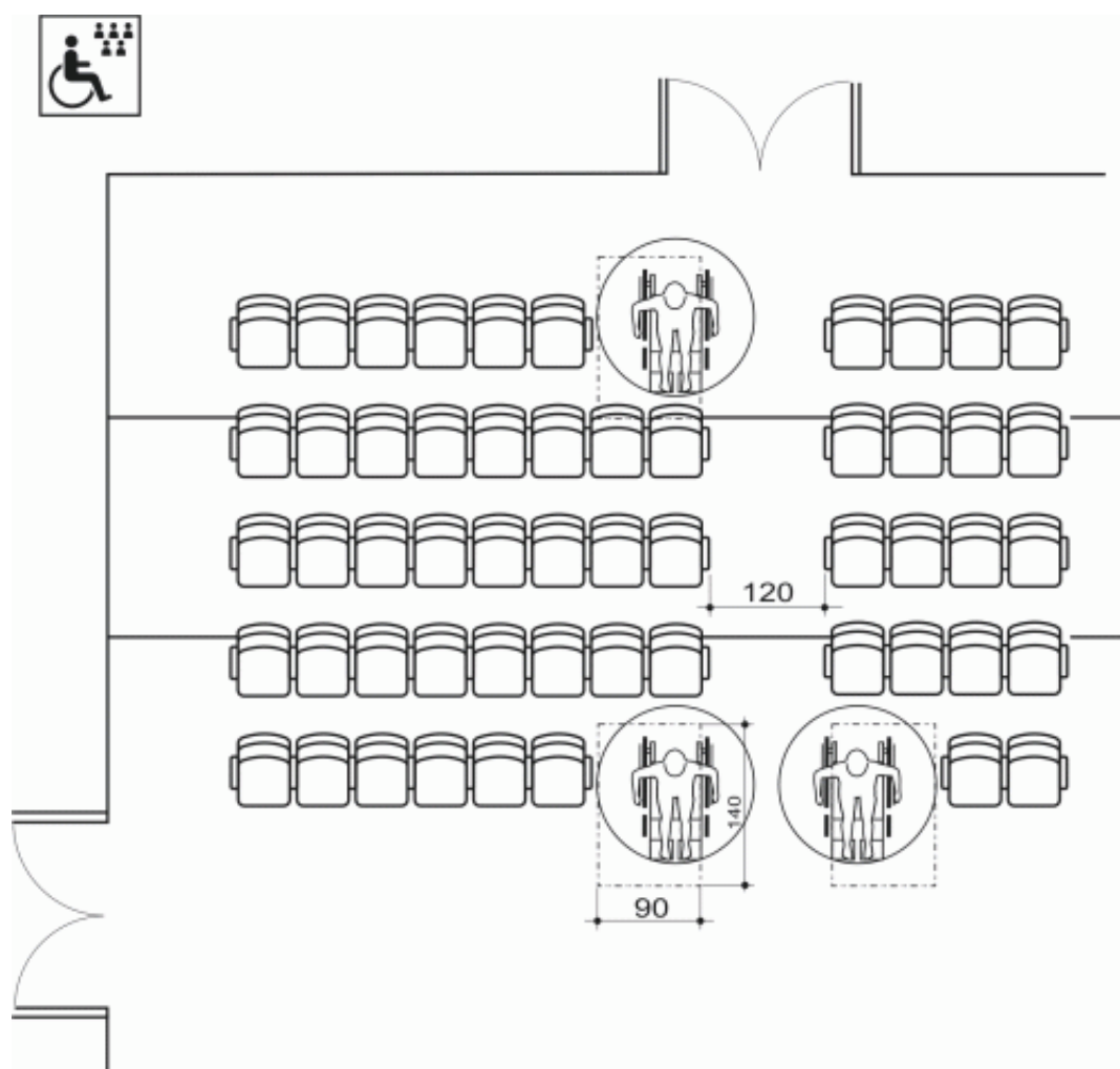
GRAFIČKI PRIKAZ BR. 28 - MJESTO U GLEDALIŠTU
