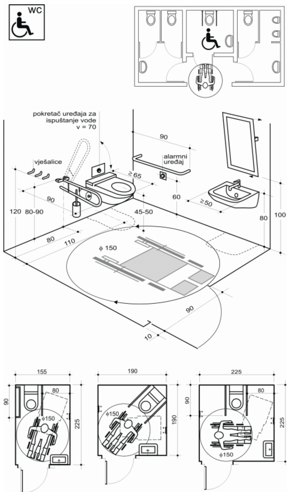
GRAFIČKI PRIKAZ BR. 15 - WC
