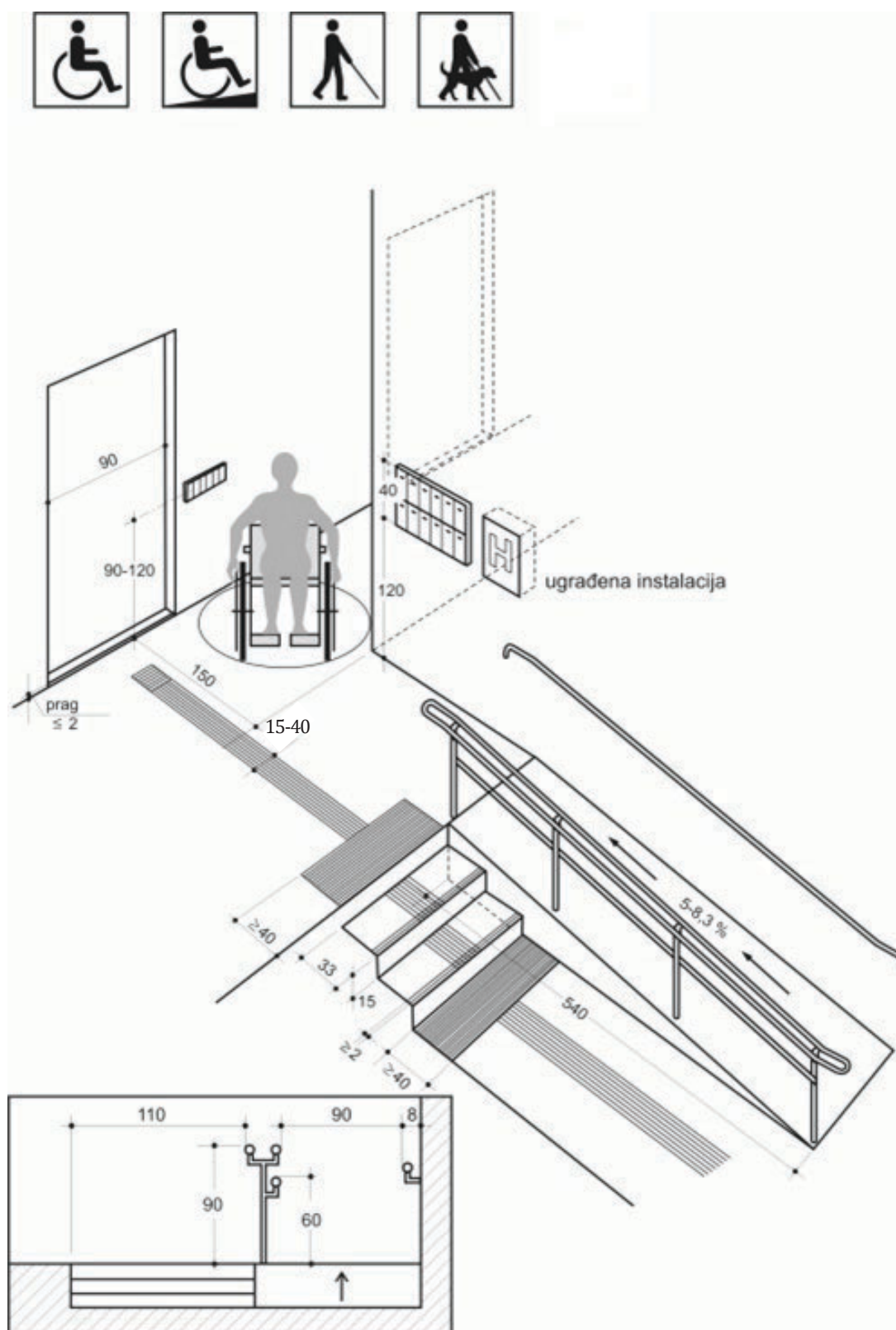
GRAFIČKI PRIKAZ BR. 14 - HODNICI
