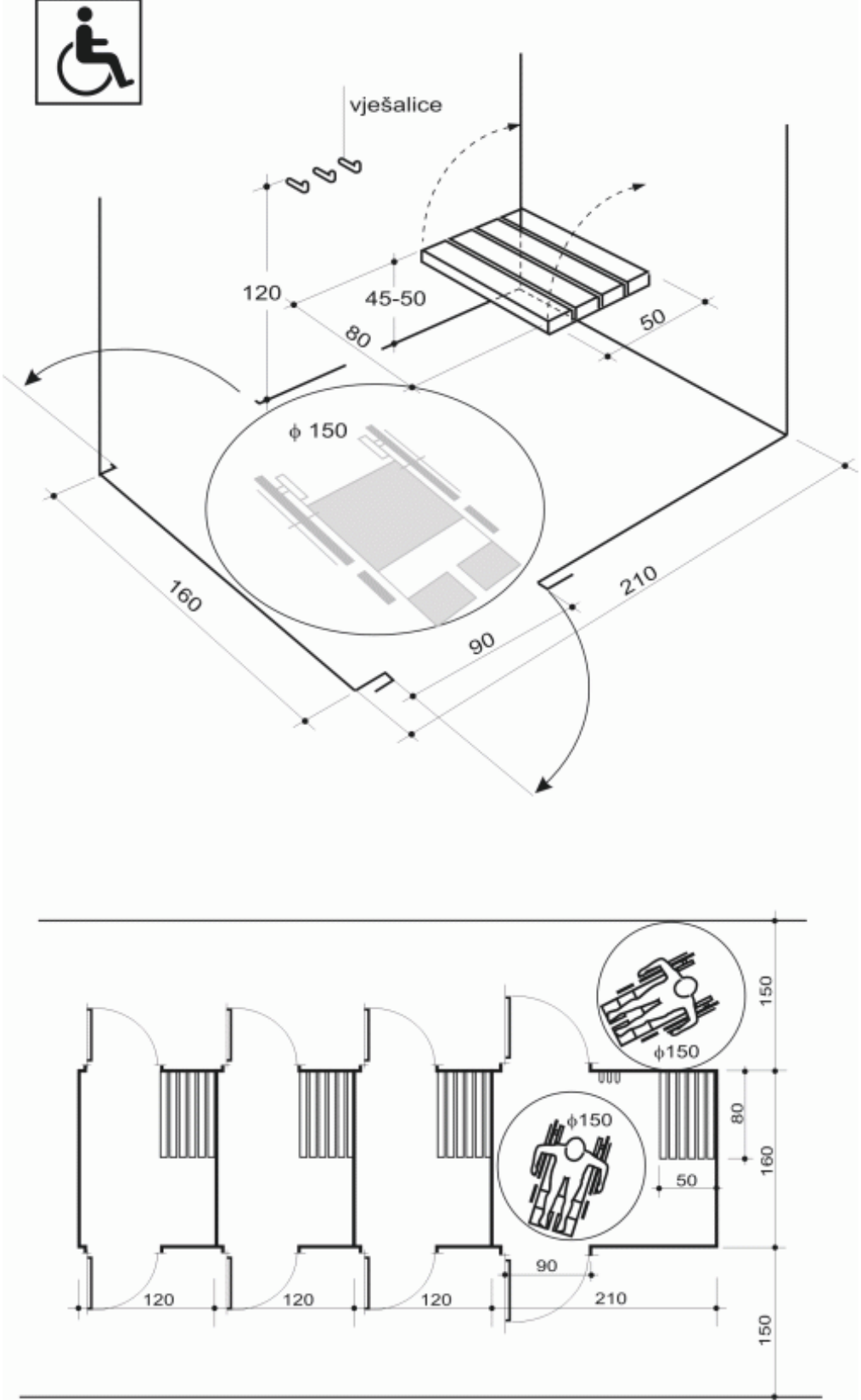
GRAFIČKI PRIKAZ BR. 24 - KABINA ZA PRESVLAČENJE
