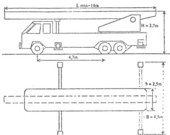
Изглед и габаритне мјере ватрогасног возила са надградњом
