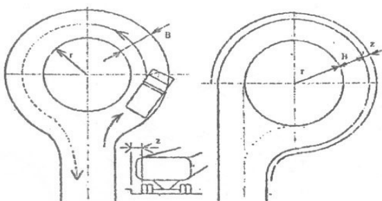
Кружне окретнице облика "О" / "Р"
